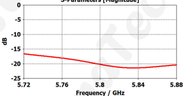
S-Parameters [Magnitude]
